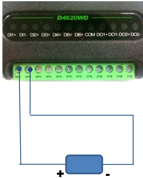
Level(Wet) 접점일 경우
